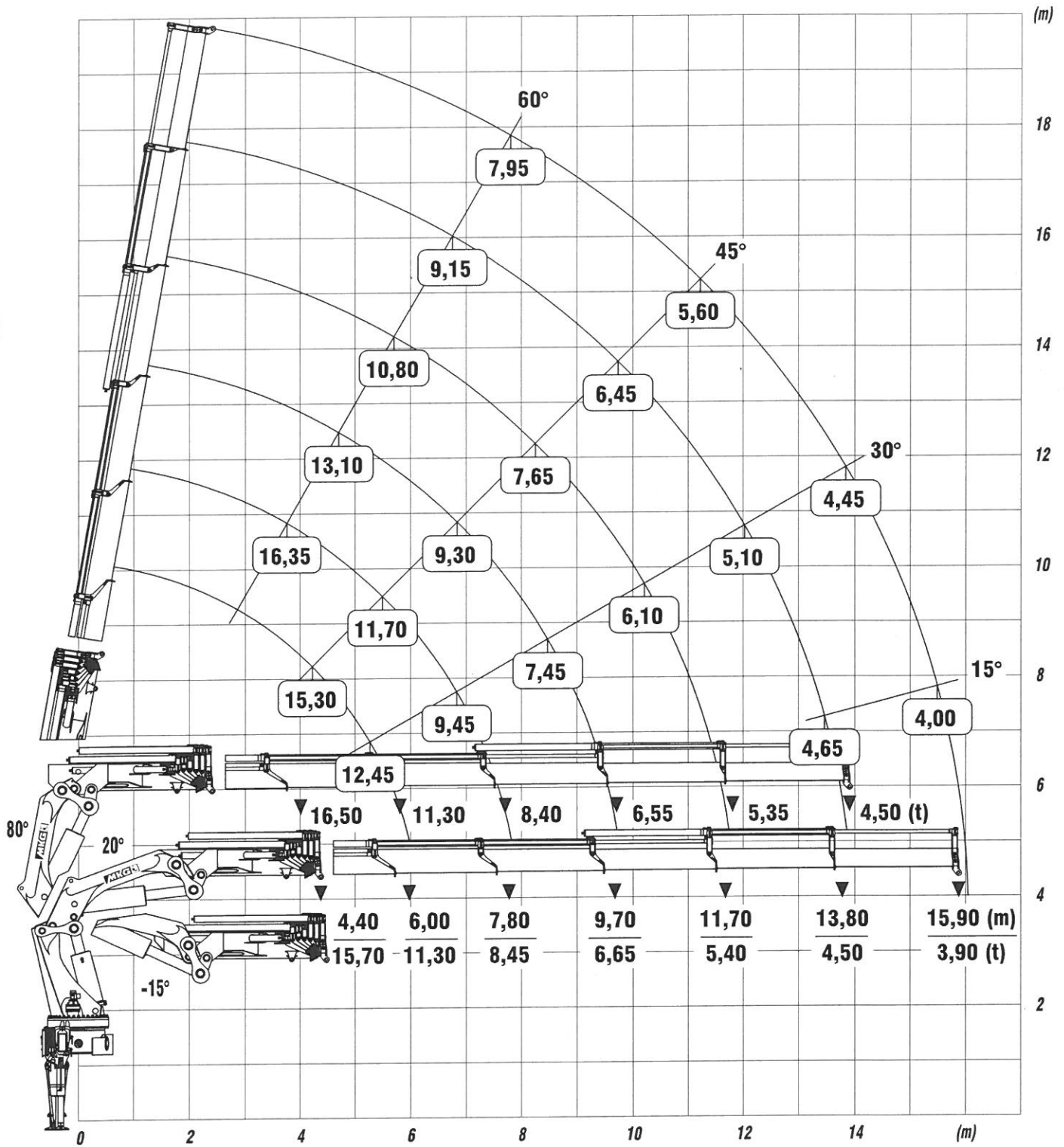
16,05 m max. hydraulische Reichweite Arm gestreckt / max. outreach (horizontal position)
